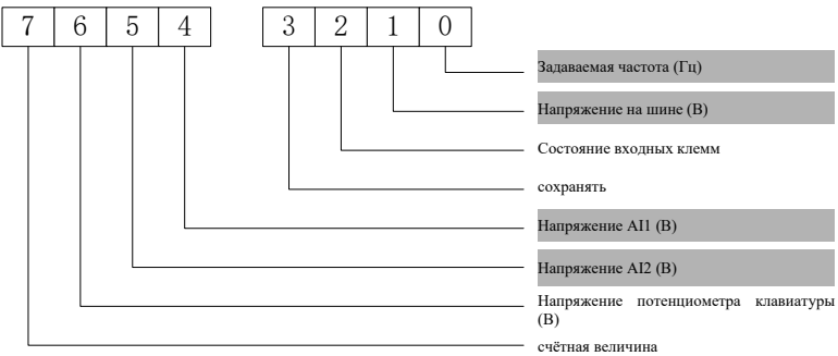
Рис. 5-7 Содержание отображения P7-05 на восьмёрке ниже
