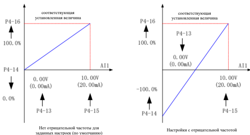
Рис. 7-13 Типичная установка кривой 1 AI1
