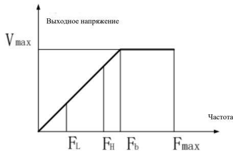
Рис. 7-1 Схема определения параметров частоты
