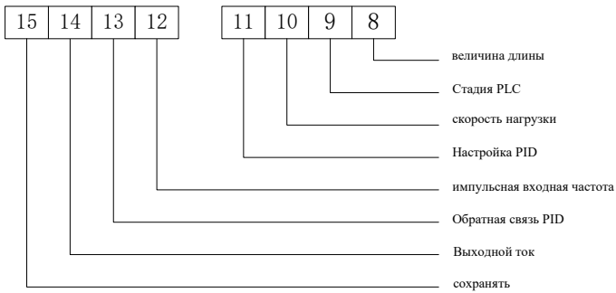
Рис. 5-8 Содержание дисплея P7-05 на восьмизначной высоте
