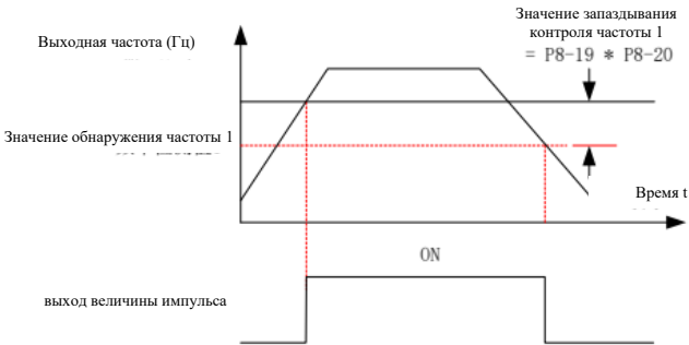
Рис. 7-15 Схема контроля уровня частоты AI
