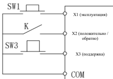
Рис. 7-12 Трехпроводный режим эксплуатации 2
