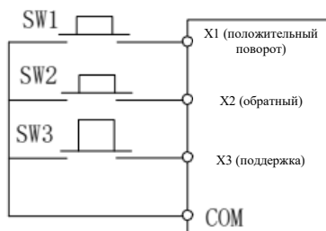
Рис. 7-11 Трехпроводный режим эксплуатации 1
